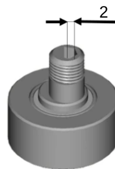
Disassamento ruote piane TIB 40 Eccentriche
